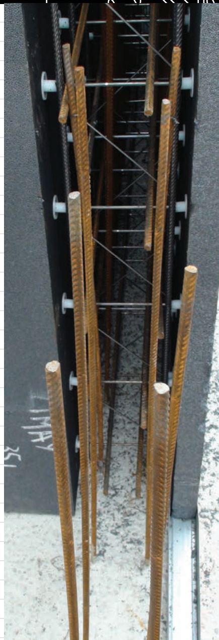
Fers d'appel
