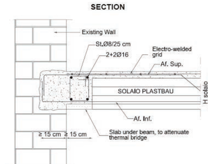
Venecia - rehabilitación del forjado
