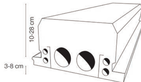
K: rango de espesor de la altura EPS (3-8 cm) H: rango de altura de la vigueta (10-28 cm) Paneles estándar
