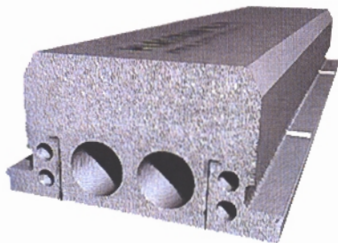
Pannello in polistirene autoportante, grazie agli inserti a Z in lamiera zincata, per la realizzazione di solai. Grazie alla sua leggerezza, la movimentazione degli elementi è estremamente agevole (Poliespanso).
